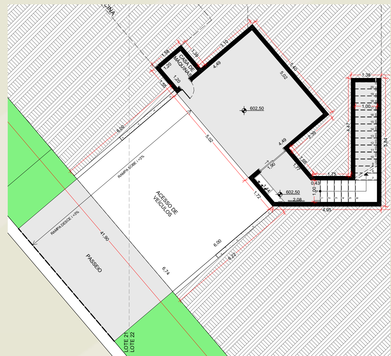
PLANTA SUBSOLO ESC.: 1:100
