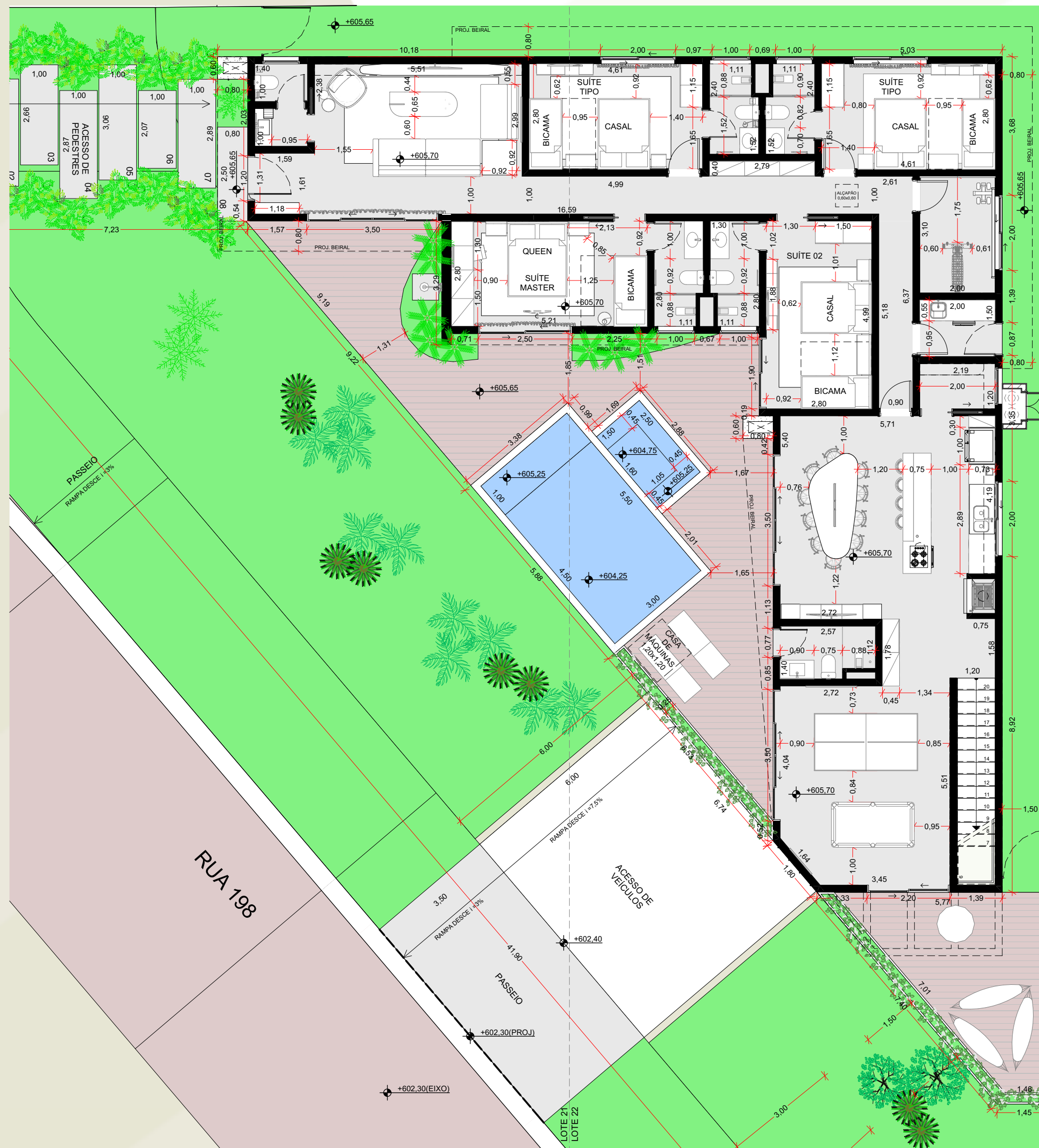
PLANTA TÉRREO ESC.: 1:100
